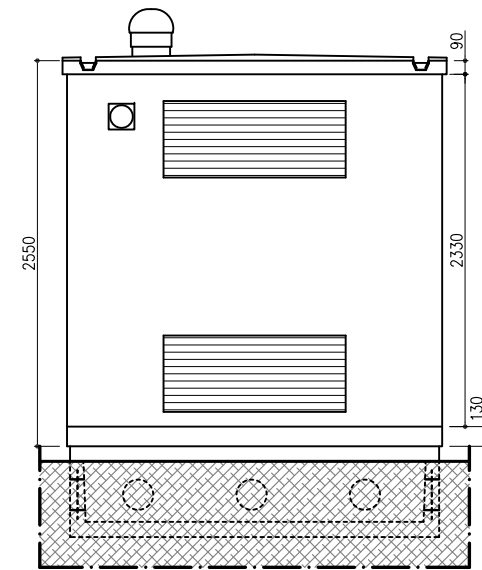
PROSPETTO B
