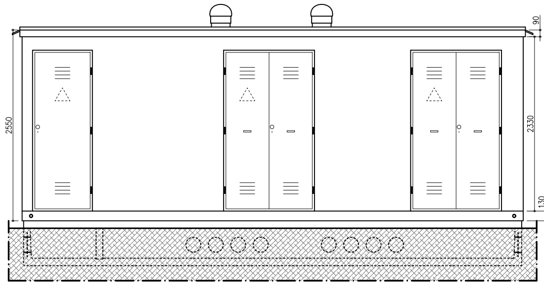
PROSPETTO A
