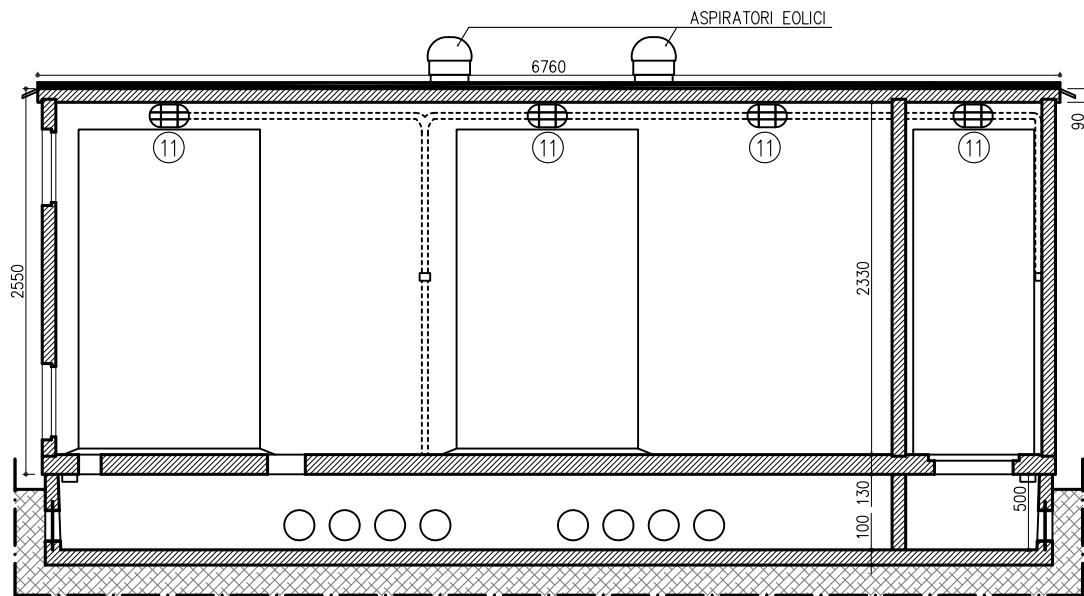
SEZIONE X-X
